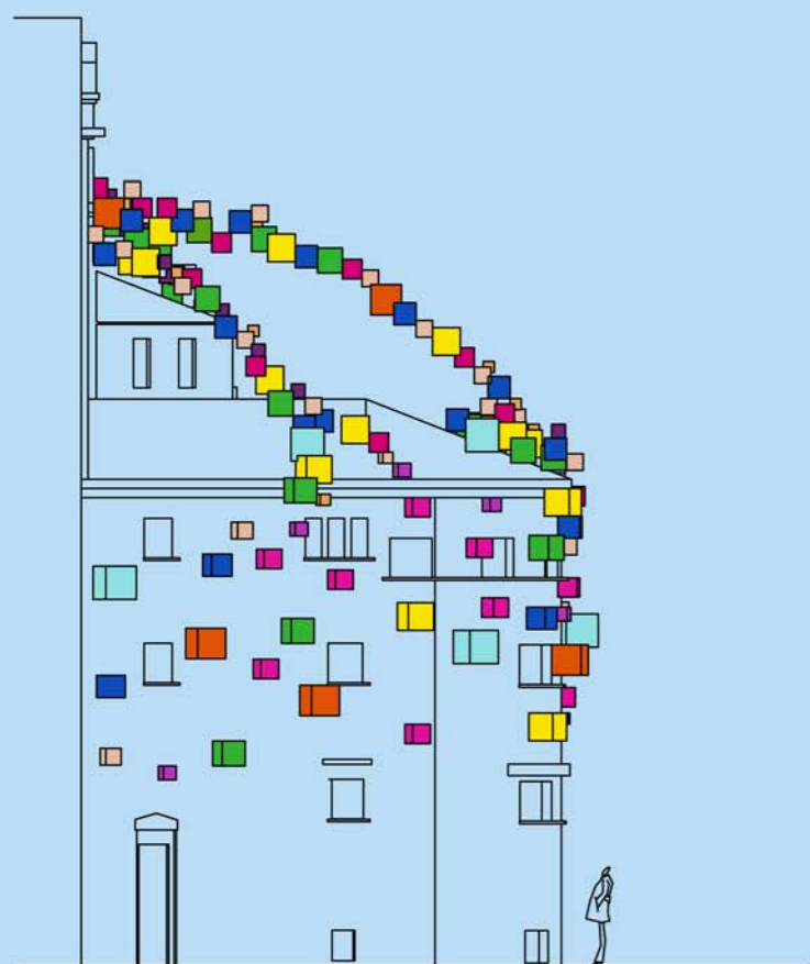
FACHADA C/ CORTES DE NAVARRA E 1:150
